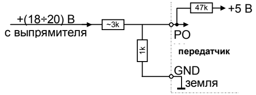
б) подключение к выпрямителю
