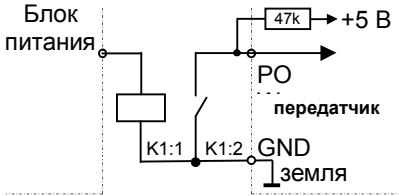
а) выход БП – реле на землю
