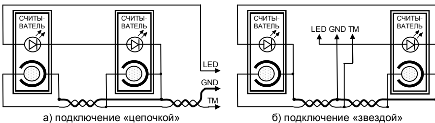
Рисунок 14 – Подключение двух считывателей
