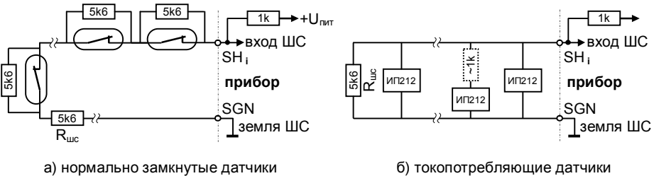
Рисунок 12 – Примеры монтажа пожарных шлейфов
