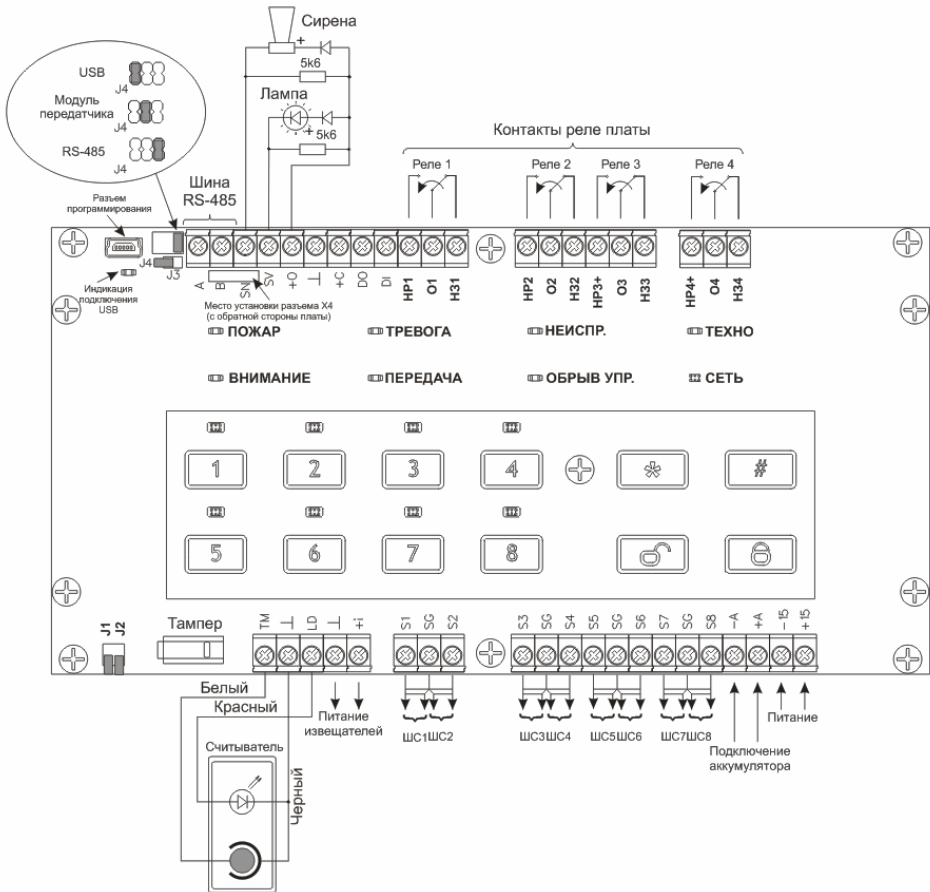
Рисунок 15 – Монтажная схема прибора
