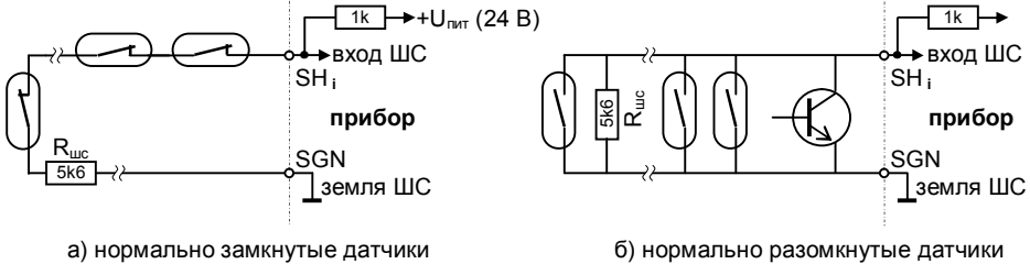
Рисунок 11 – Примеры монтажа охранных шлейфов
