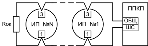
Рис.2 Типовая схема подключения извещателей к ППКП со знакопостаным ШПС
