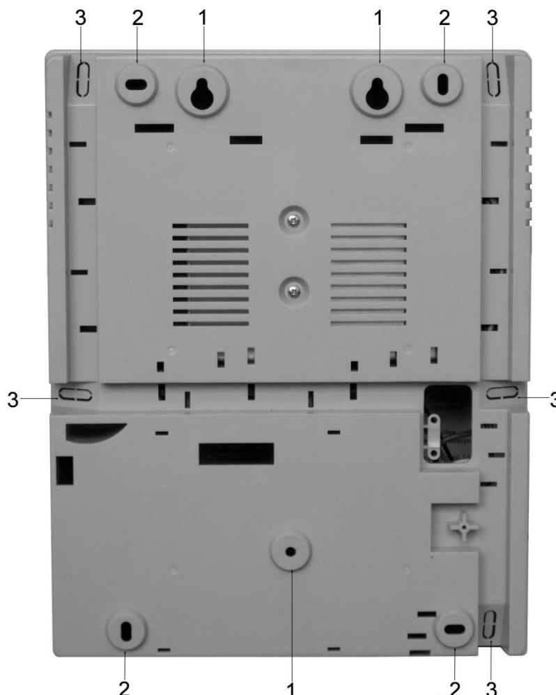
Рисунок 7. Монтажные отверстия
