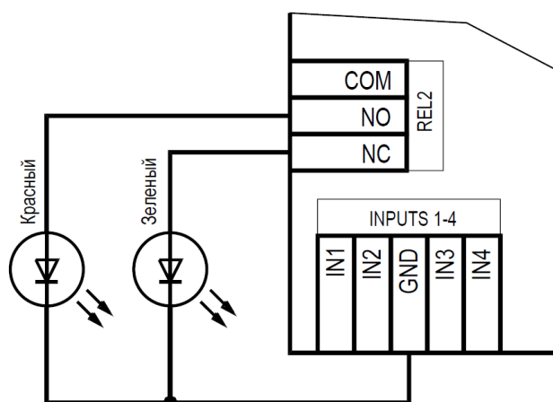
Рисунок 6. Подключение светодиодов
