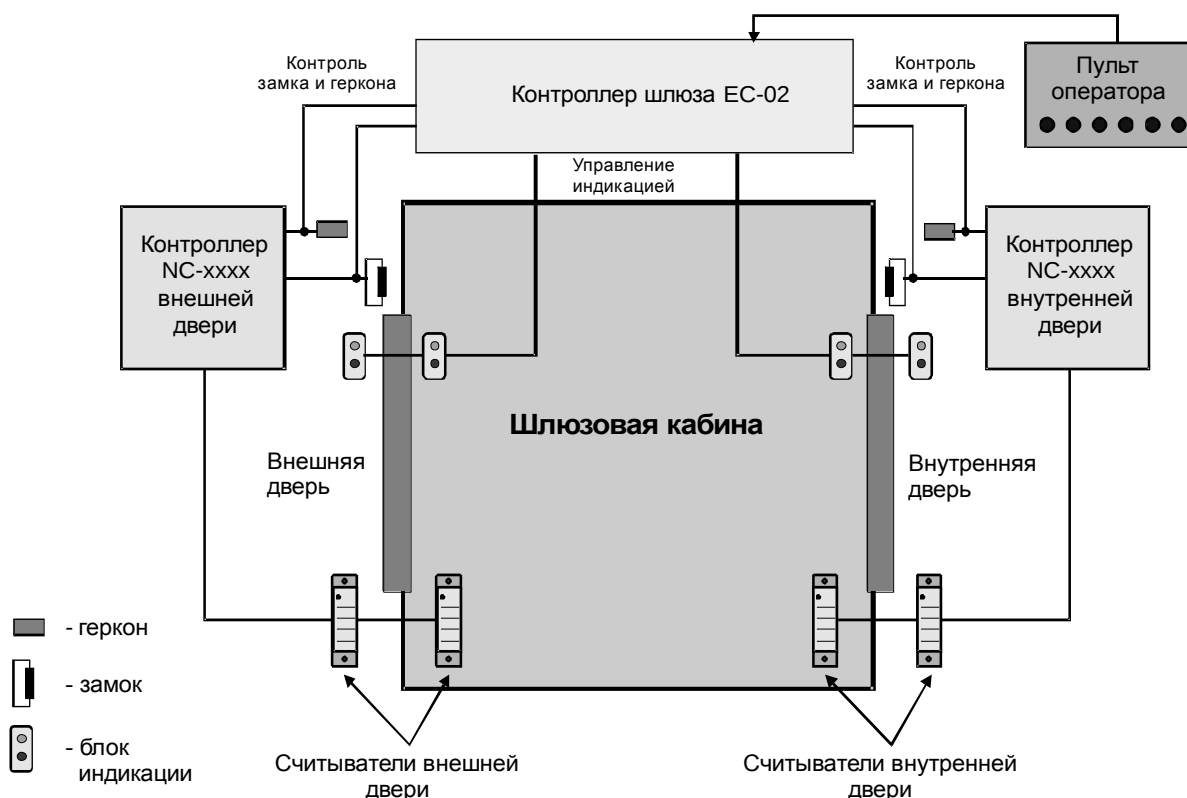
Рисунок 3. Оборудование шлюзовой кабины
