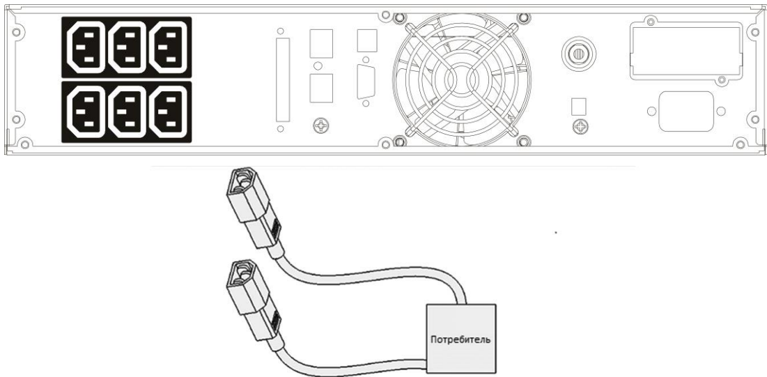
Рис. 6 Подключение оборудования к выходу ИБП
