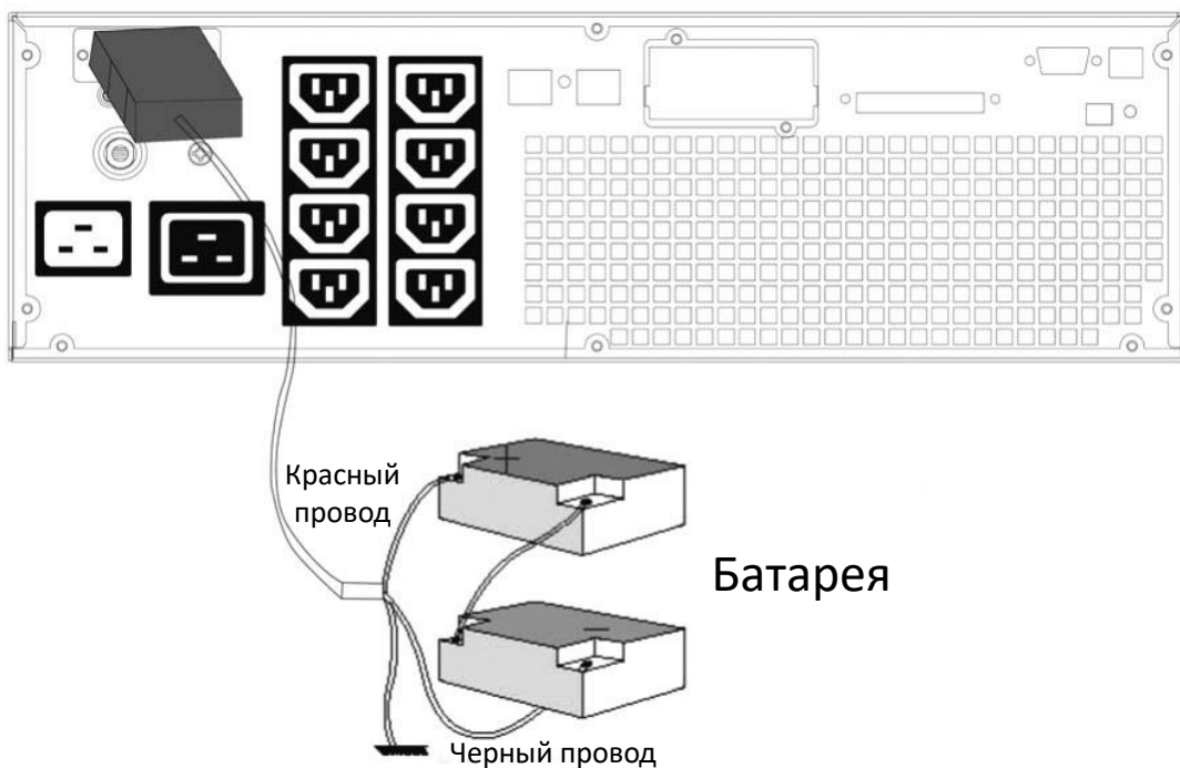
Рис. 7 Подключение аккумуляторной батареи для увеличения времени автономной работы
