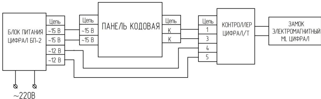
Рисунок А.4 Стандартная схема подключения панели кодовой с контроллером замка ЦИФРАЛ/Т
