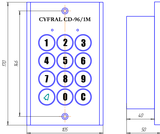
Рисунок А.2 Габаритные и установочные размеры панели кодовой ЦИФРАЛ CD-
