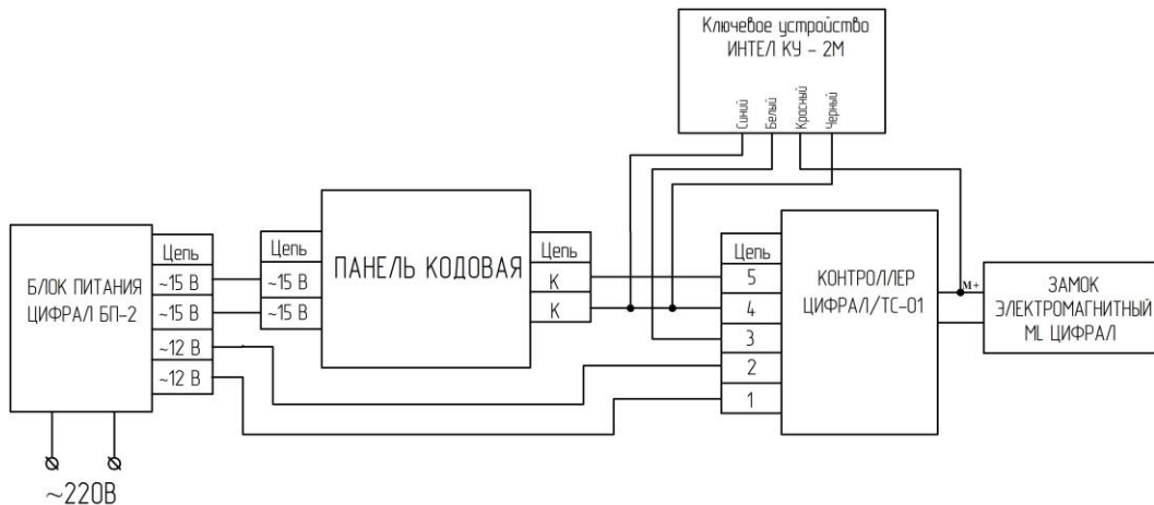
Рисунок А.5 Схема подключения панели кодовой с контроллером замка ЦИФРАЛ/ТС-01 и устройством ключевым ИНТЕЛ КУ-2М
